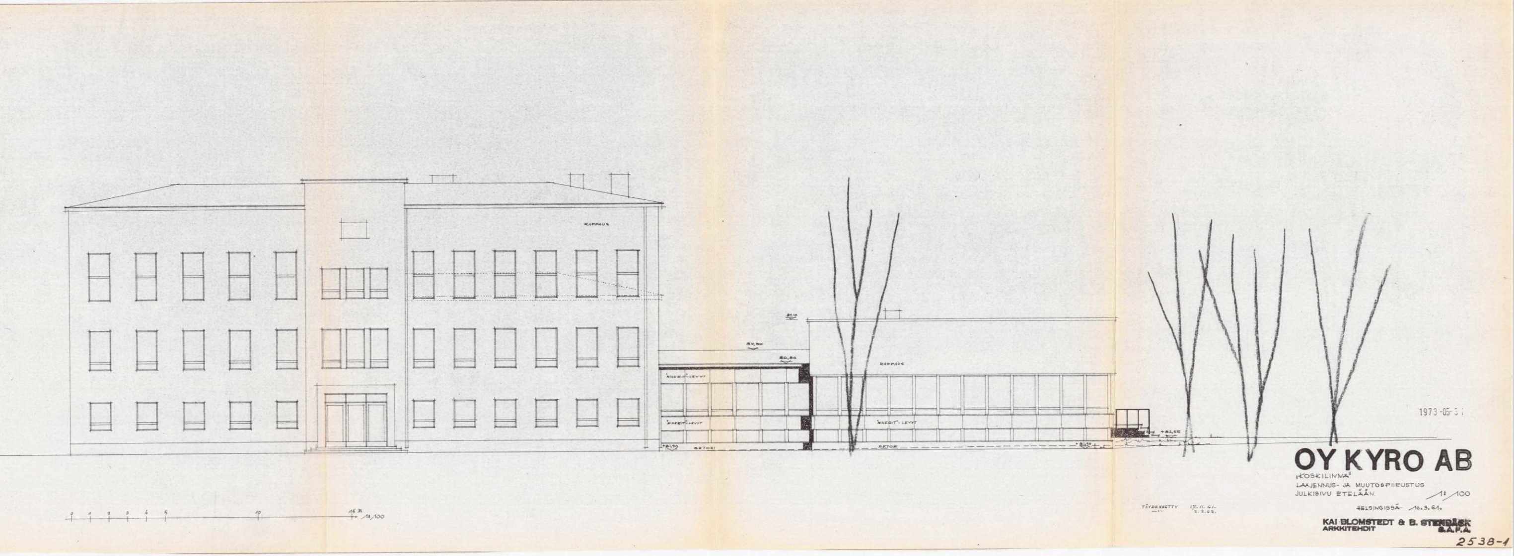
1961 julkisivut etelään ja länteen (ei mittakaavassa)
