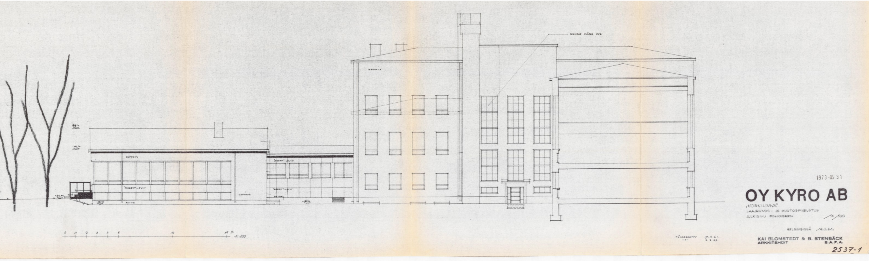
1961 julkisivut pohjoiseen ja itään (ei mittakaavassa)
